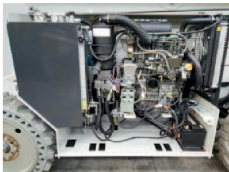
3válcový naftový motor Yanmar, 18 kW
